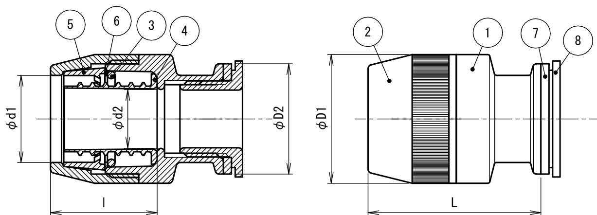
断面図
